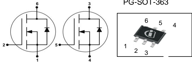
PG-SOT-363
